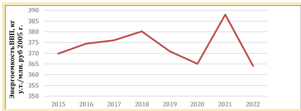
Рисунок 4 - График изменения энергоемкости Беларуси
